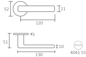
3095 5S Q | Puxador Door handle | Poignée
