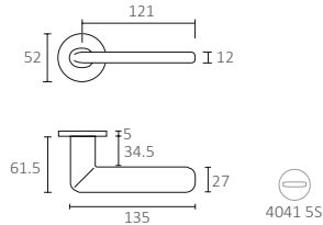
3098 5S Q | Puxador Door handle | Poignée
