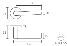
1967 5S Q | Puxador Door handle | Poignée
